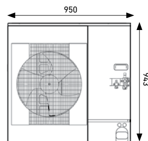
Unidad exterior 8 kW
