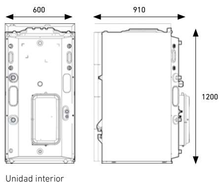
Unidad interior
