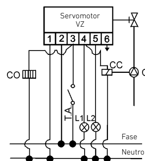
Conexiones eléctricas
