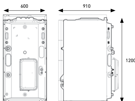
Unidad interior
