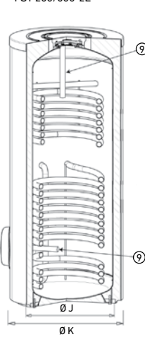
FST 200/500-2E
