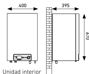
Unidad interior
