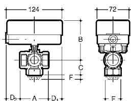
Válvula de zona motorizada de 3 y 2 vías
