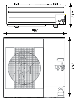
Unidad exterior 8 kW
