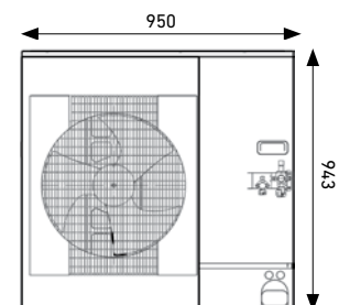
Unidad exterior 8 kW
