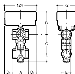
Válvula de zona motorizada con detentor
