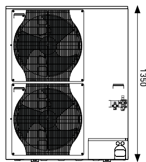
Unidad exterior 11 y 16 kW
